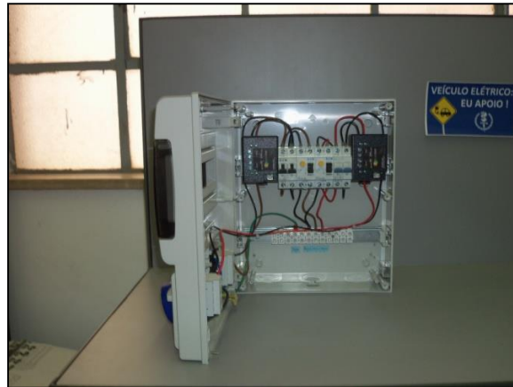
Figuras 4A e 4B. Vistas frontal e interna do painel de recarga dos carros elétricos
