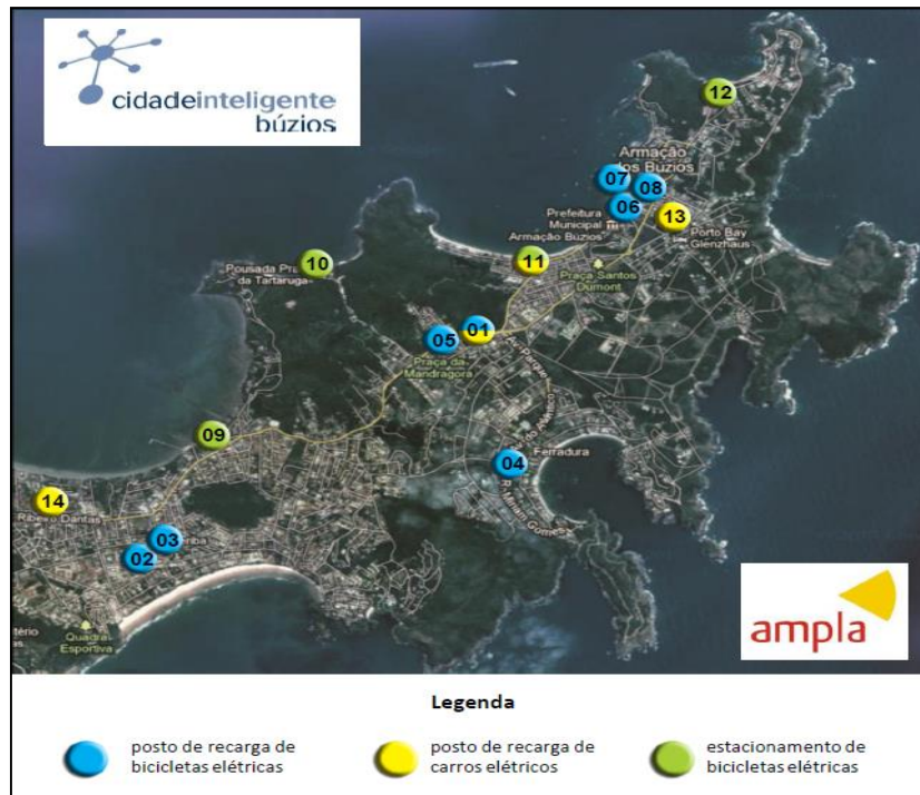
Figura 1. Infraestrutura de recarga de veículos elétricos do projeto
