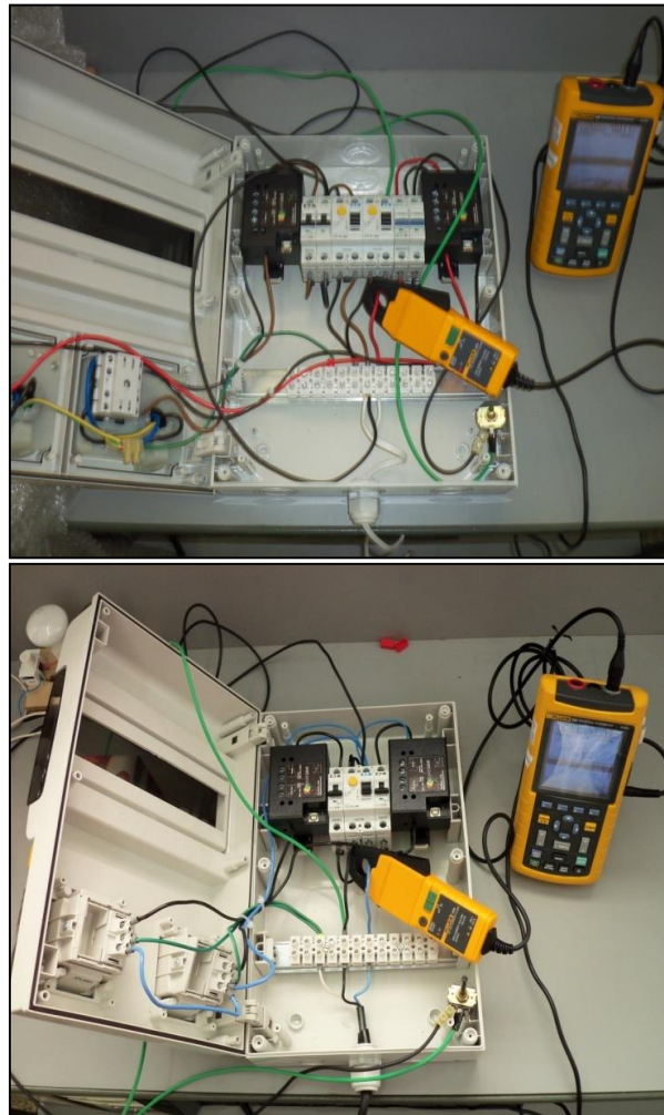
Figuras 7A e 7B. Painel dos carros e das bicicletas: ensaio de verificação da atuação dos DR_{(s)}
