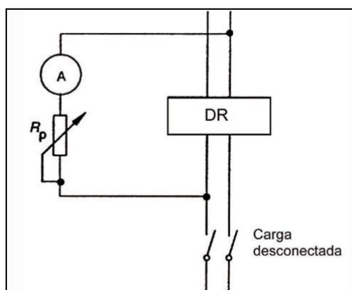
Figura 6. Esquema para ensaio de verificação da atuação do DR (S)
